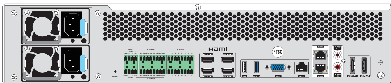
TNVR-641H背面 端子配置図
