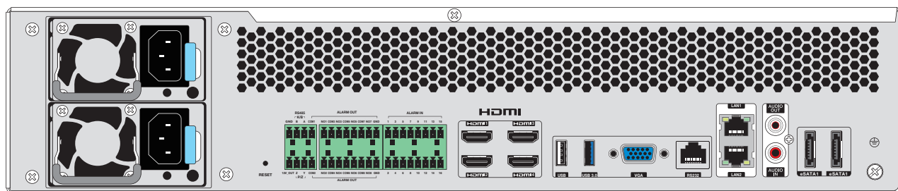
TNVR-324H背面 端子配置図
