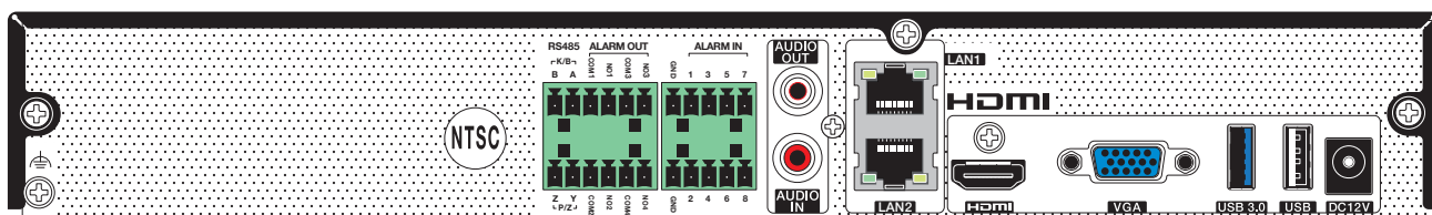
TNVR-802H背面 端子配置図
