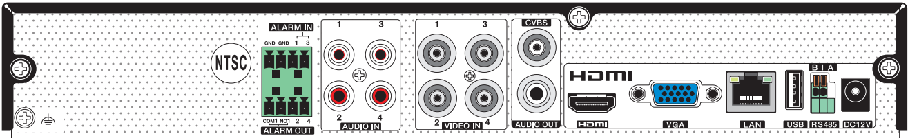
TXVR-401H背面図
