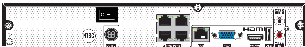
TNVR-401HP背面図
