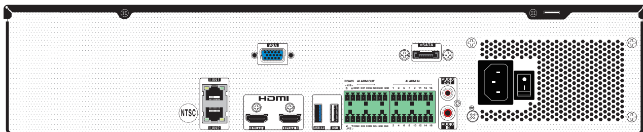
TNVR-321H背面 端子配置図
